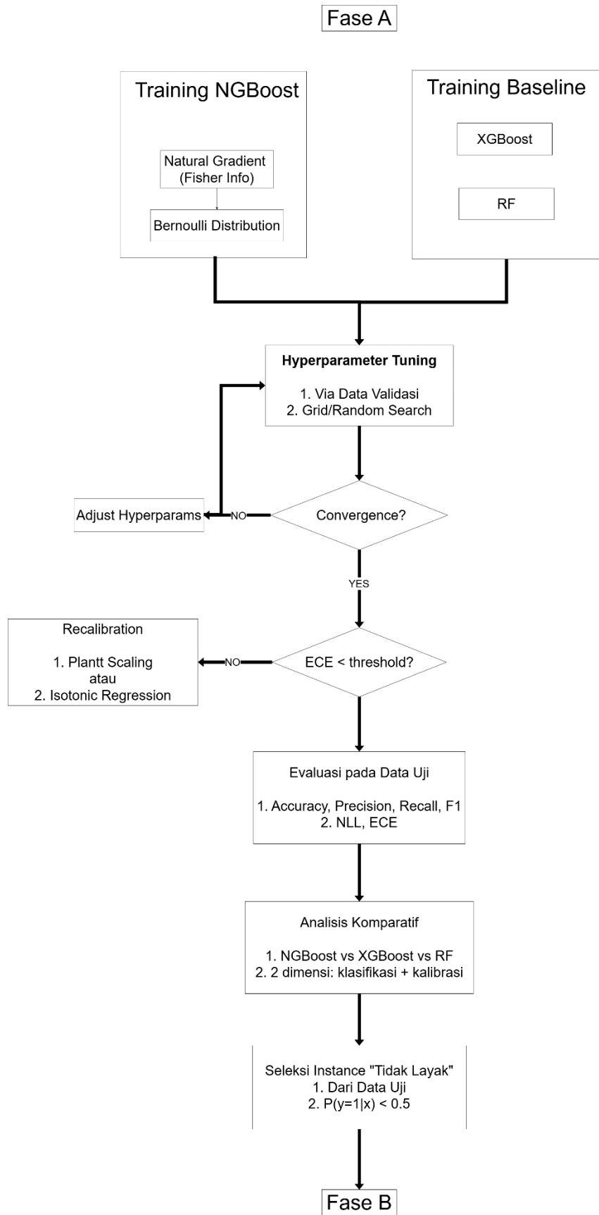
Gambar 3.2 Alur Diagram Pemodelan Fase A (Sumber: Peneliti).
