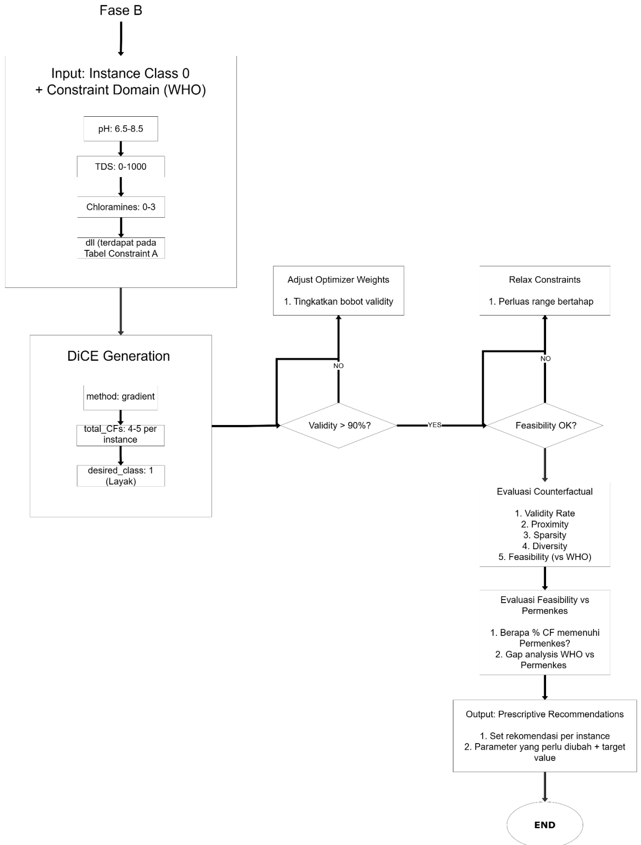
Gambar 3.3 Alur Diagram Pemodelan Fase B (akhir) (Sumber: Peneliti).
