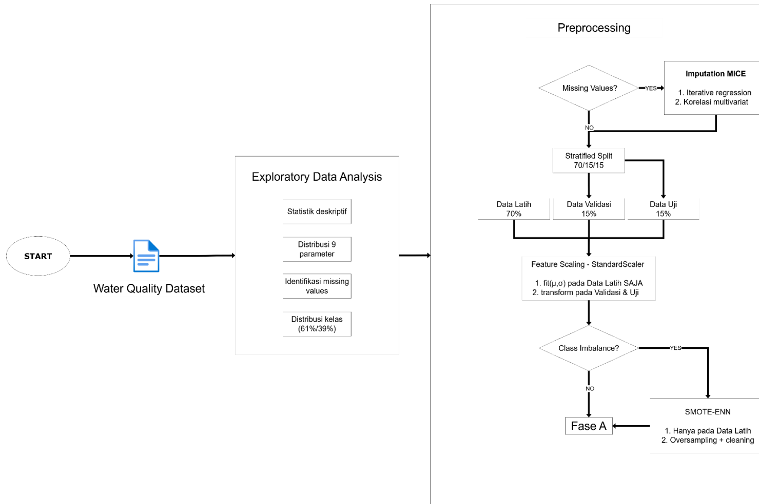
Gambar 3.1 Alur Diagram Pemodelan Fase Awal (Sumber: Peneliti).
